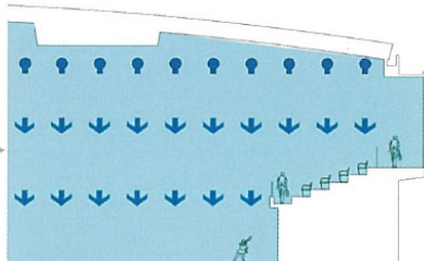
全体空調方式の場合
